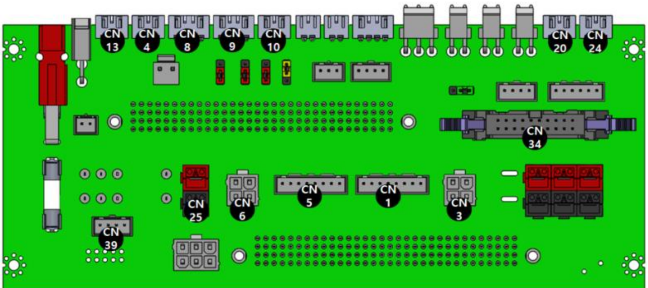
<그림 3-18> Interface Ports on BackLink
