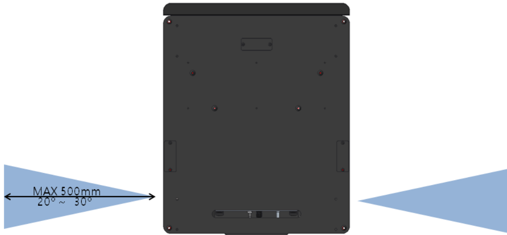
<그림 3-5> Angle and maximum distance of Ultrasonic Sensors
