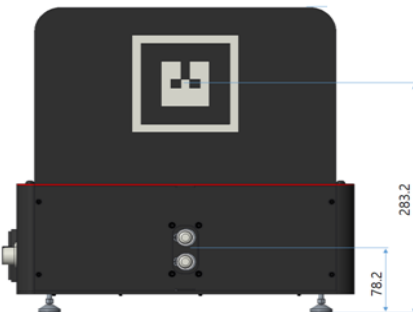
<그림 2-2> Physical Dimensions of TETRA-DSV
