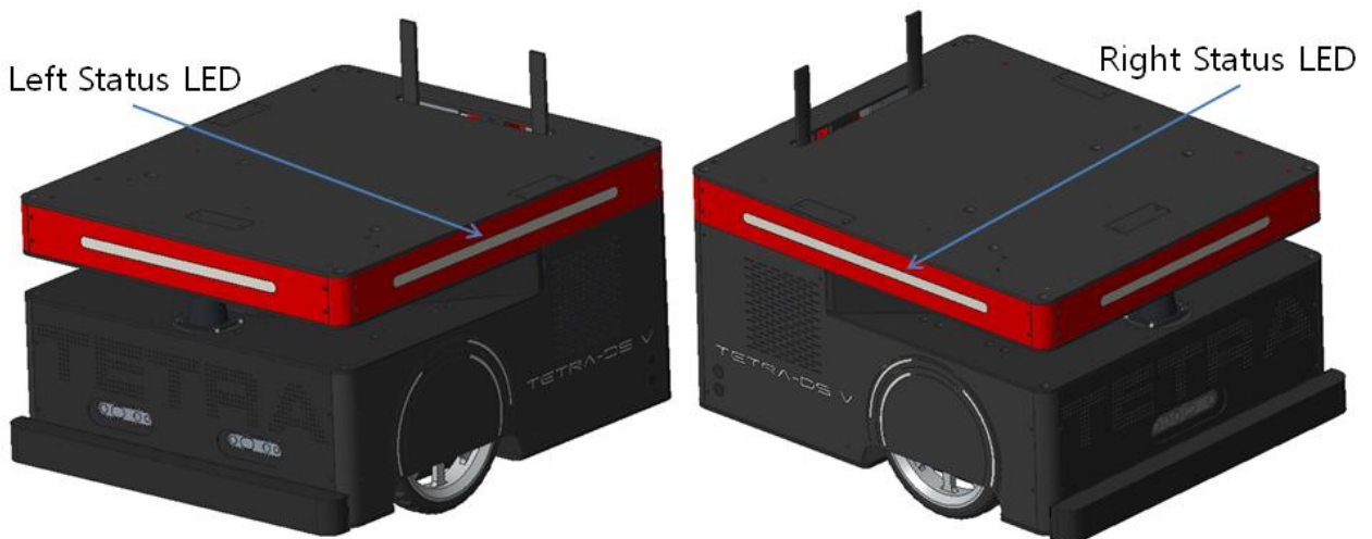
<그림3-8> Side Status LED
