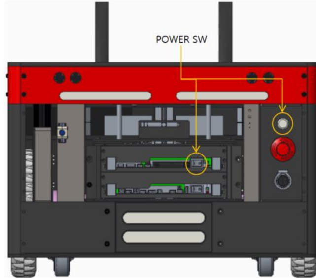
<그림 3-9> Main Power Switch
