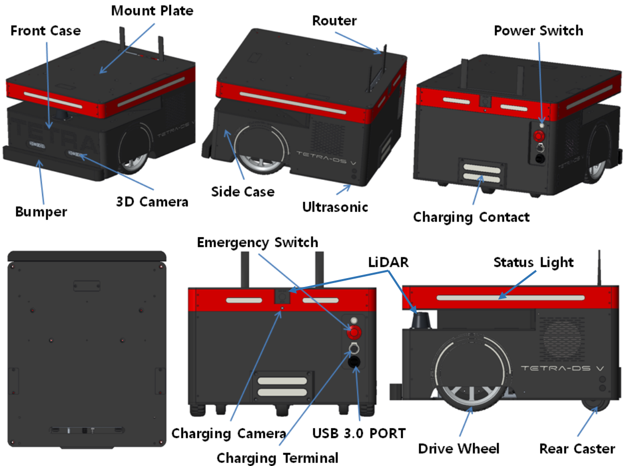
<그림 2-1> Components Layout of TETRA-DSV
