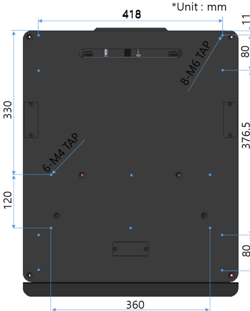
<그림 2-3> Dimensions of Taps on Mount Plate
