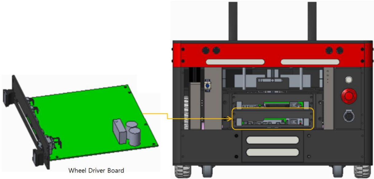
<그림 3-16> Components Layout of Drive Board
