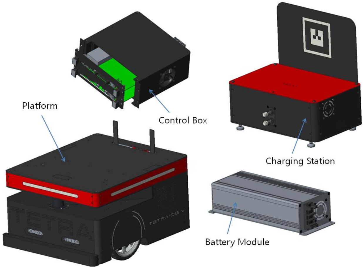
<그림 1-3> TETRA-DSV Package
